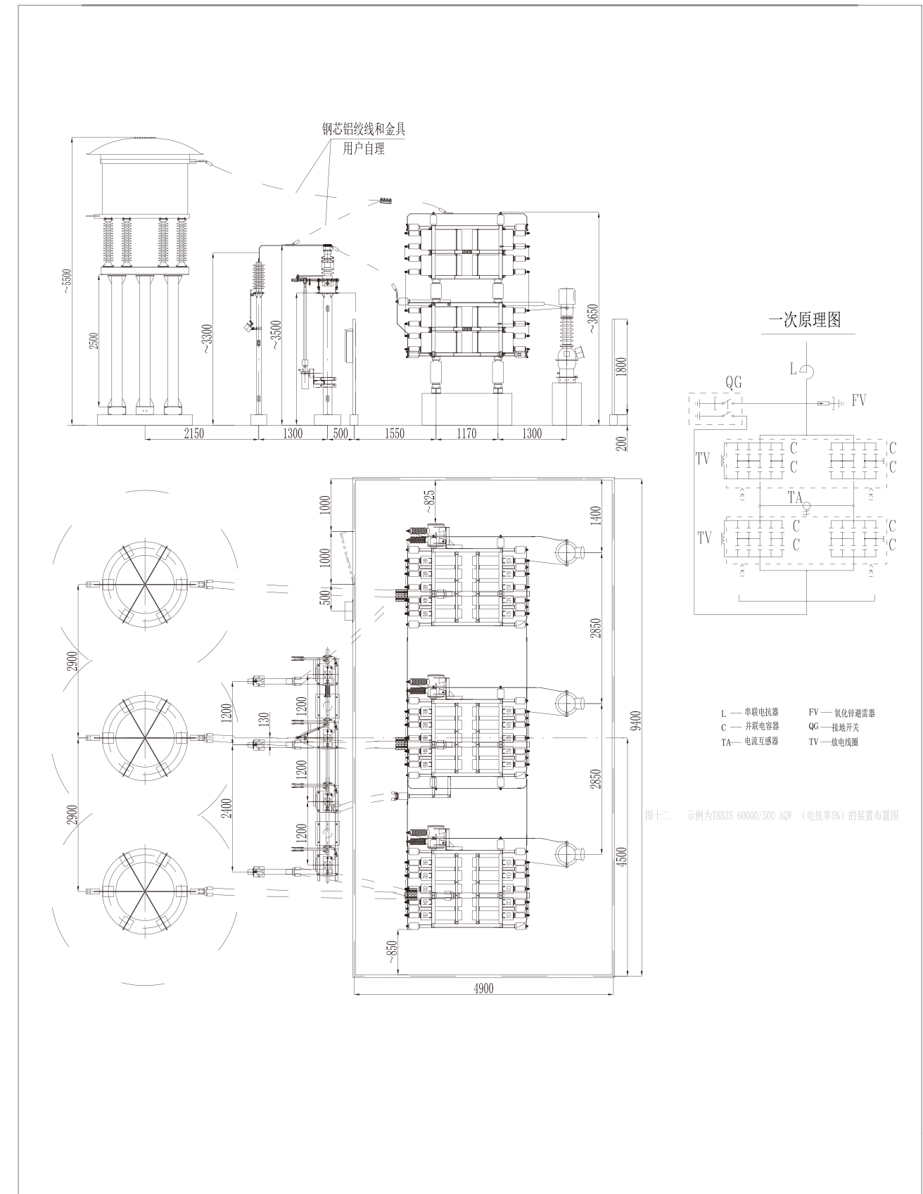
图十二 示例为 TBB35-60000/500-AQW（电抗率 5%）的装置布置图
