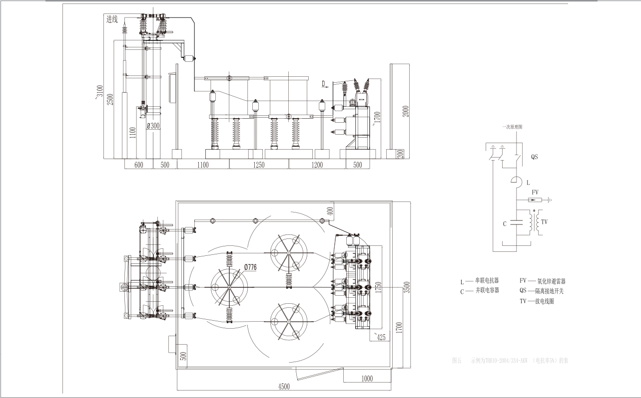
图六 示例为 TBB10-4008/334-AKW（电抗率5%）的装置布置图
